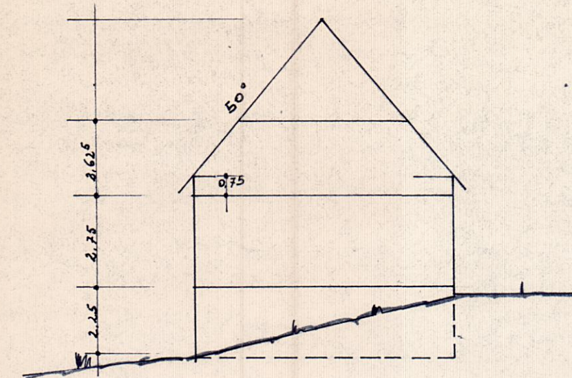
BAUTYP A
